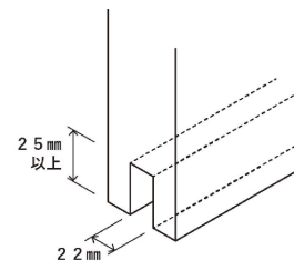
▲下部振止溝の加工寸法
