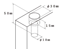
▲上部吊金具の加工寸法
